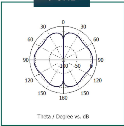
6 GHz
